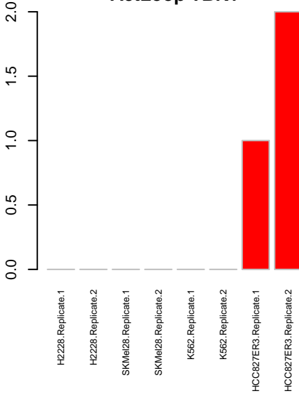
ActLoop TBK1
