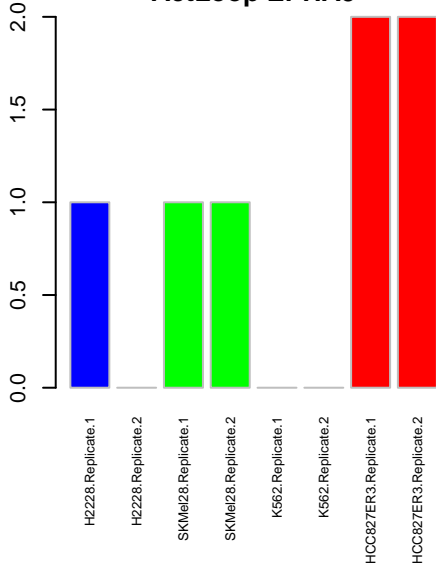
ActLoop EPHA5
