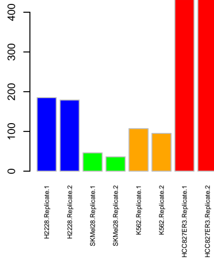
NWK EGFR
