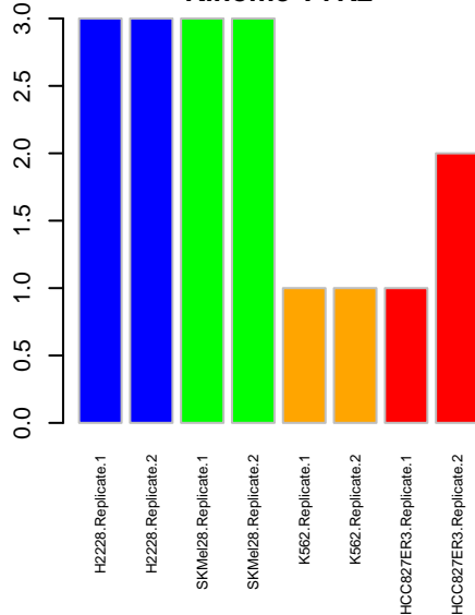
Kinome TYK2
