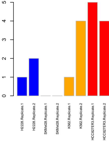
PSP CDK2
