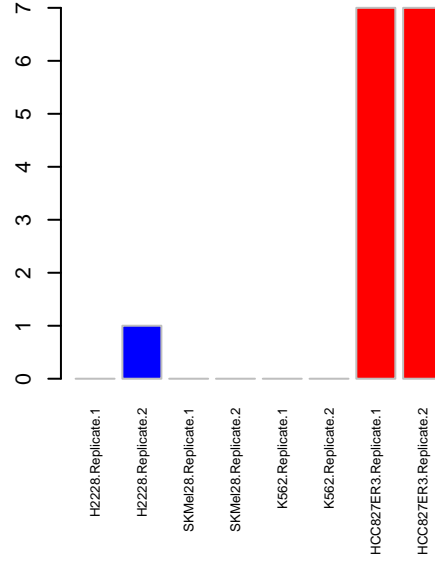
Kinome ERBB4
