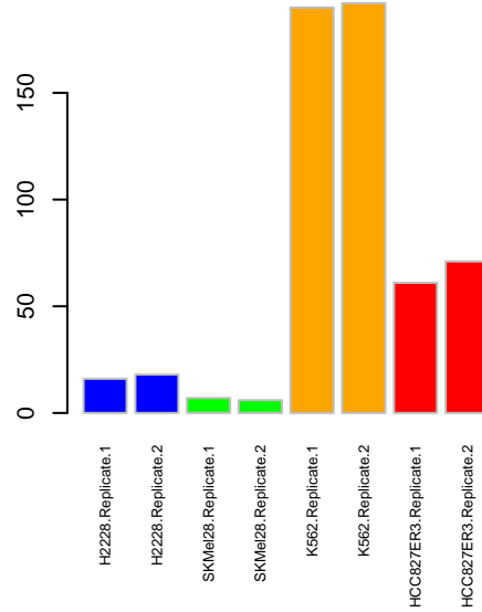
PSP FYN
