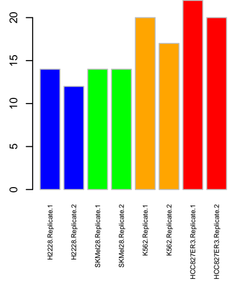
NWK MAP2K3
