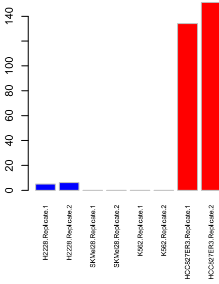
Kinome EGFR
