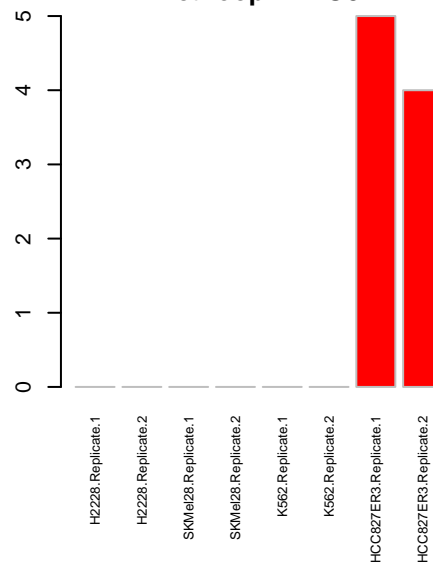
ActLoop TYRO3
