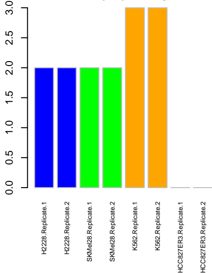
Kinome HIPK3
