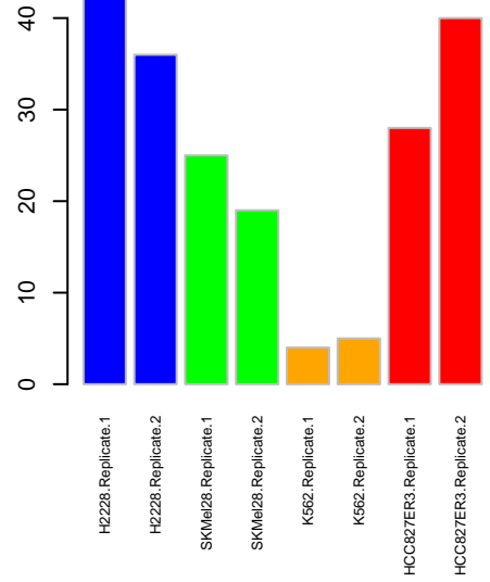
Kinome PTK2
