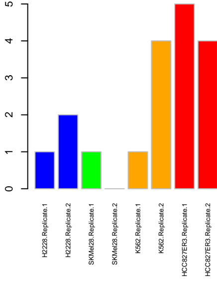
PSP CDK1
