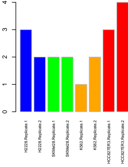
Kinome RIPK2
