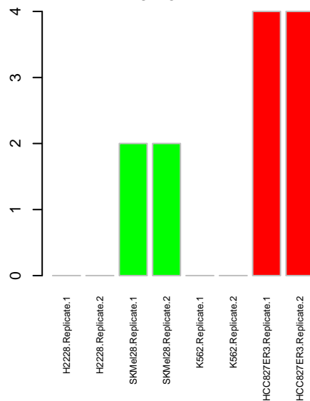
Kinome MAPK12
