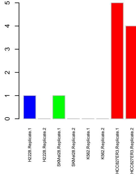
PSP JAK1
