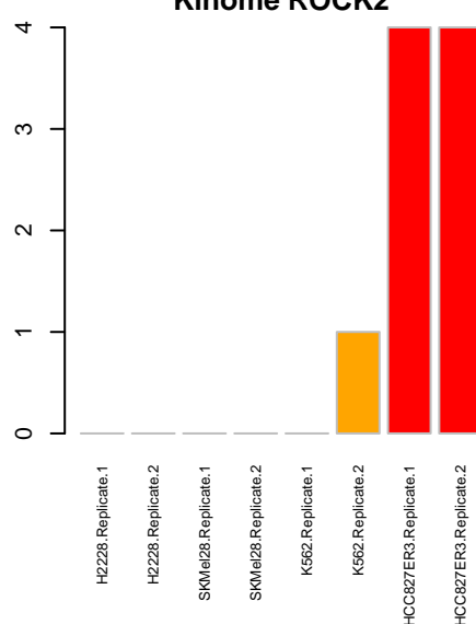
Kinome ROCK2
