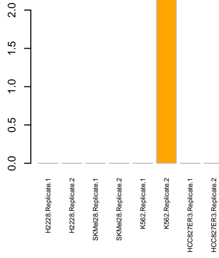
InKA PRKCD
