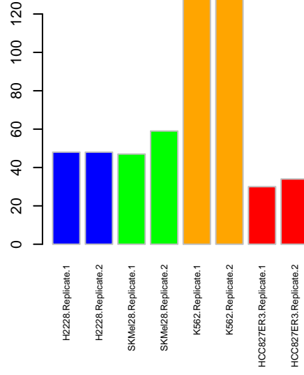
Kinome CDK1
