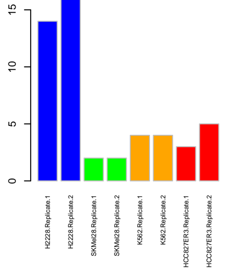
NWK INSRR
