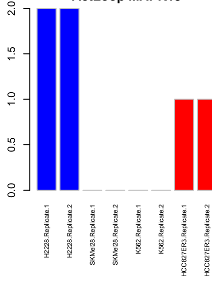
ActLoop MAPK13
