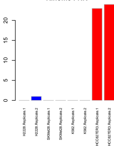
Kinome FRK
