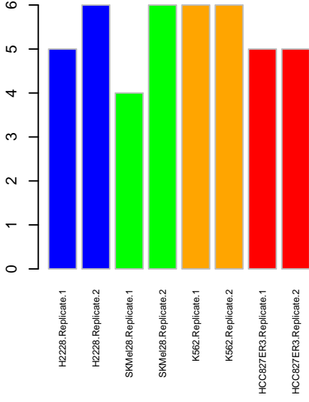
ActLoop HIPK2
