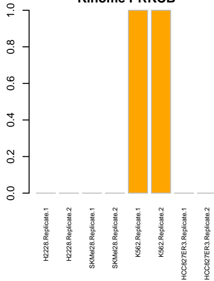
Kinome PRKCB
