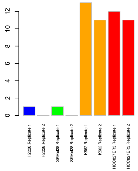
PSP JAK3
