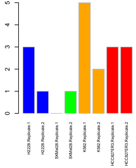
PSP KDR
