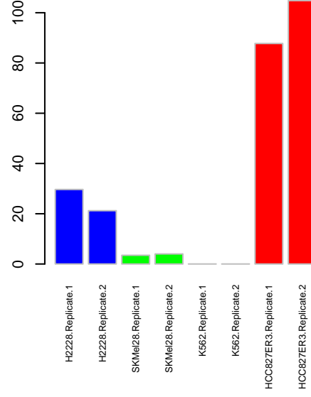
InKA EPHA2
