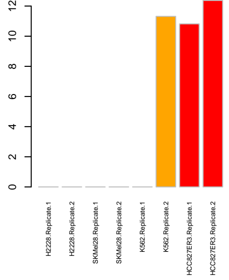
InKA TTK
