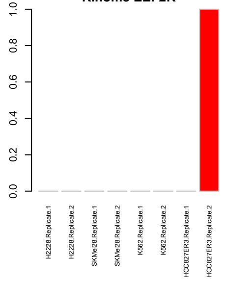
Kinome EEF2K
