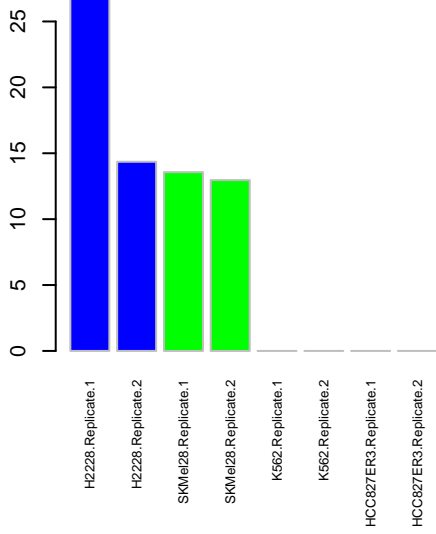
InKA INSR
