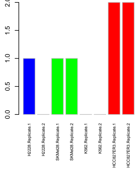
Kinome EPHA4
