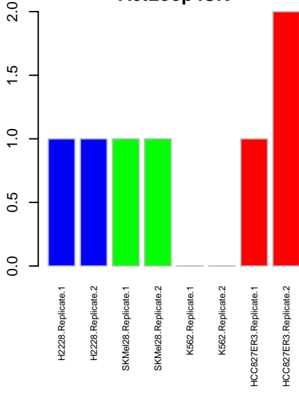
ActLoop ICK
