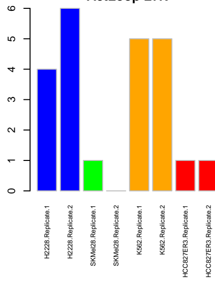
ActLoop LYN
