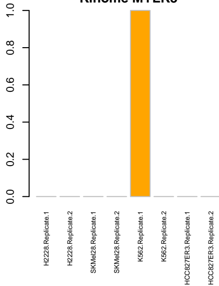
Kinome MYLK3
