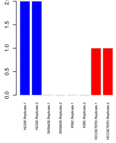
Kinome MAPK13
