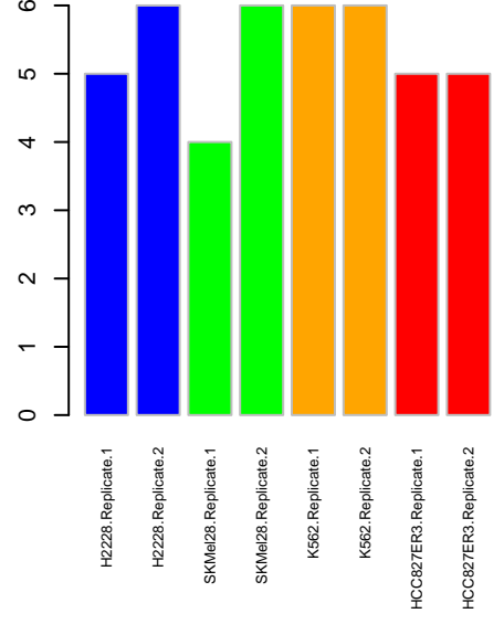
ActLoop HIPK1
