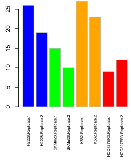
PSP MAP2K4
