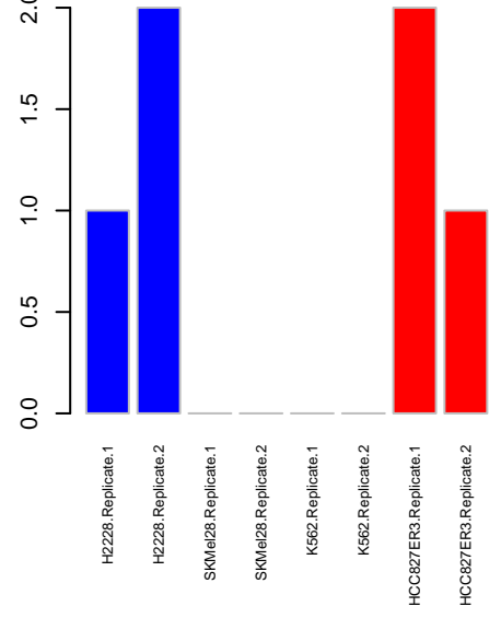
Kinome PRKCA
