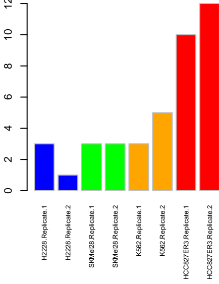
NWK MST1R
