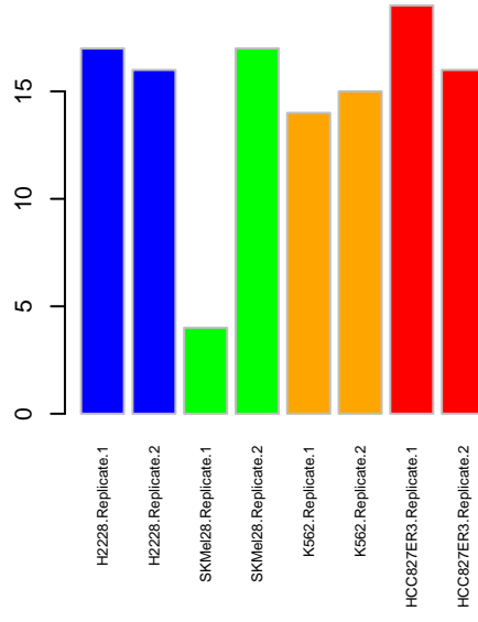
ActLoop GSK3B
