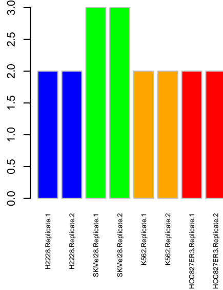
Kinome DYRK2
