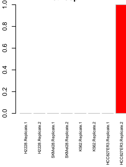
ActLoop TYK2
