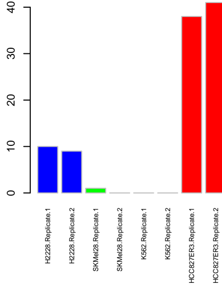
NWK AKT1
