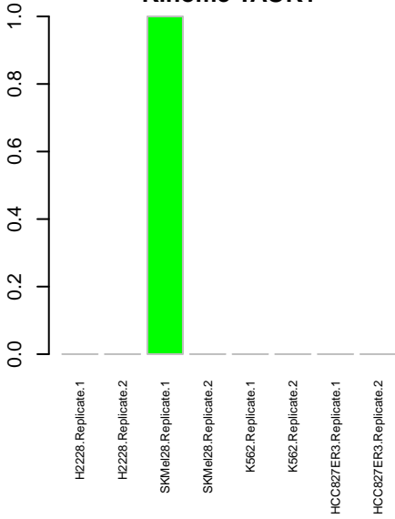
Kinome TAOK1
