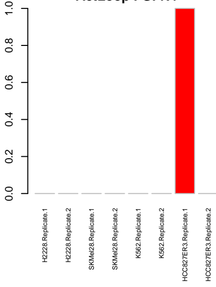
ActLoop FGFR4
