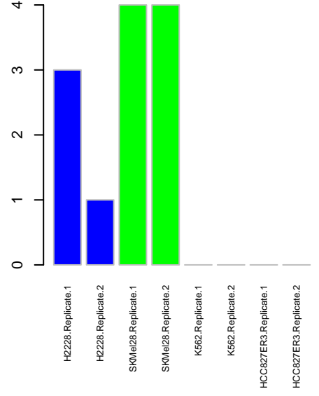
ActLoop INSR
