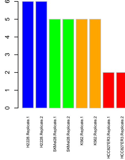
Kinome LCK
