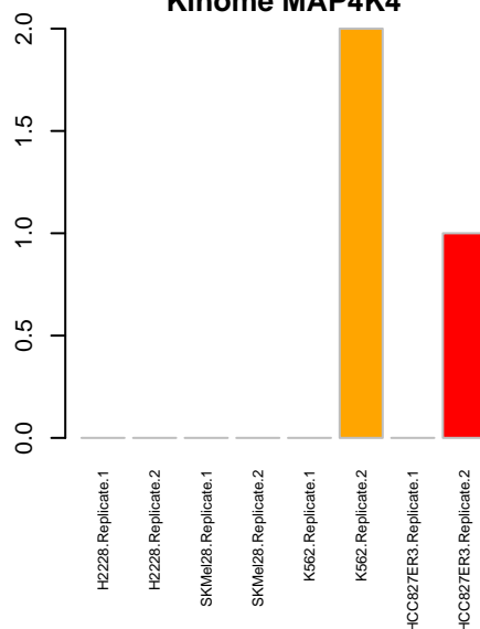
Kinome MAP4K4
