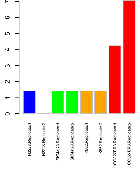
InKA MAPK10
