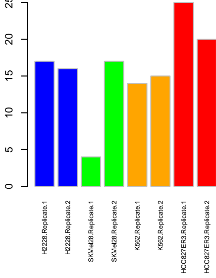
PSP GSK3B
