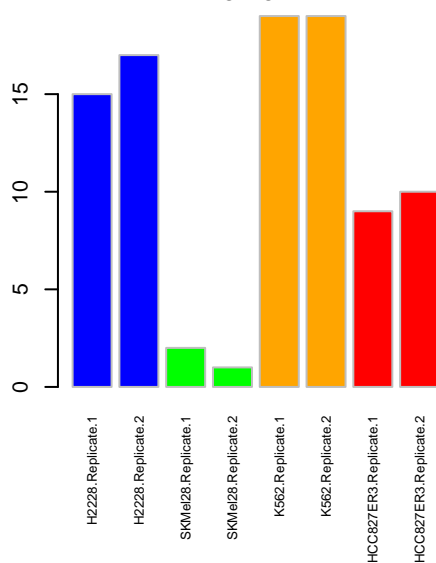
Kinome LYN
