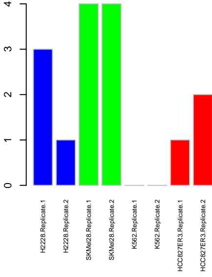
NWK IGF1R
