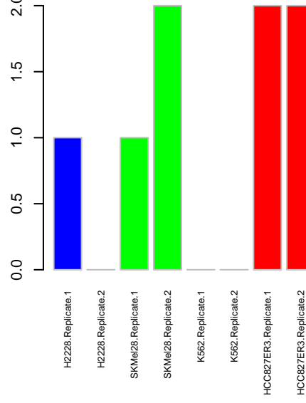
Kinome EPHA3
