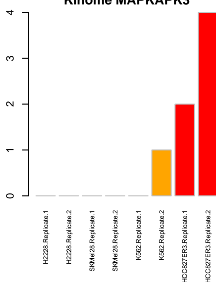
Kinome MAPKAPK3
