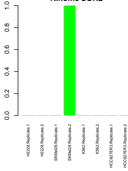
Kinome DDR2
