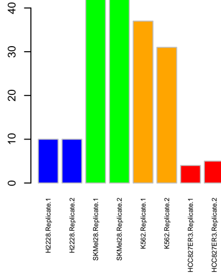
ActLoop MAPK1
