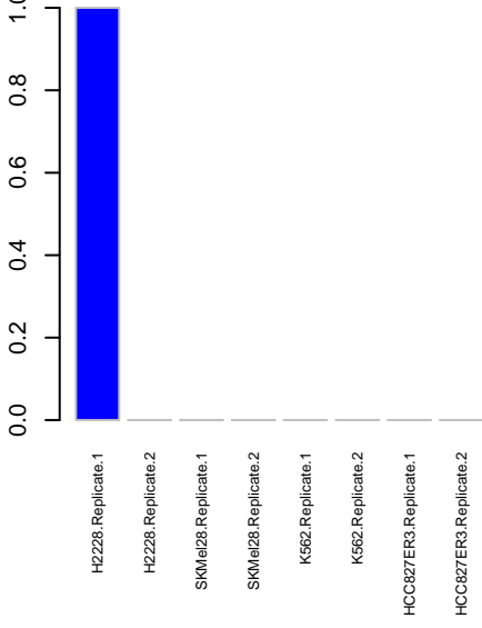
Kinome FGFR1
