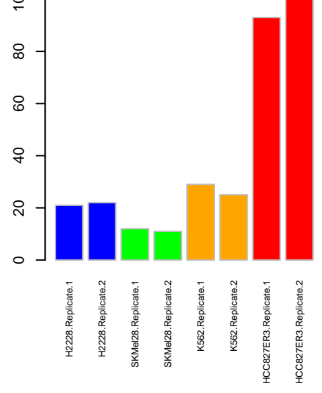
NWK MAPK3
