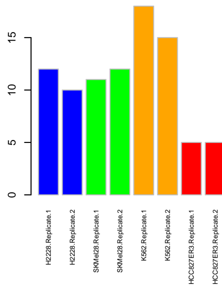
Kinome DYRK1A
