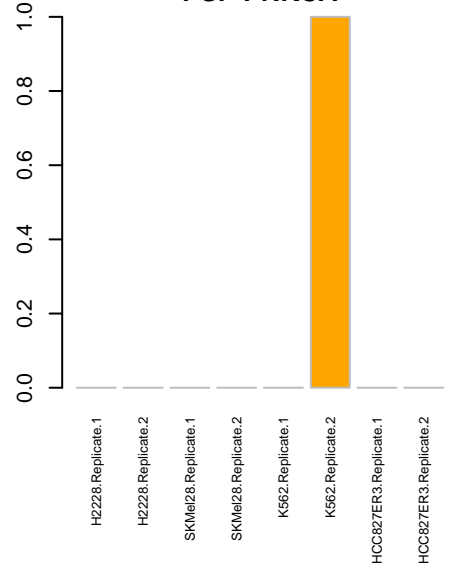
PSP PRKCA
