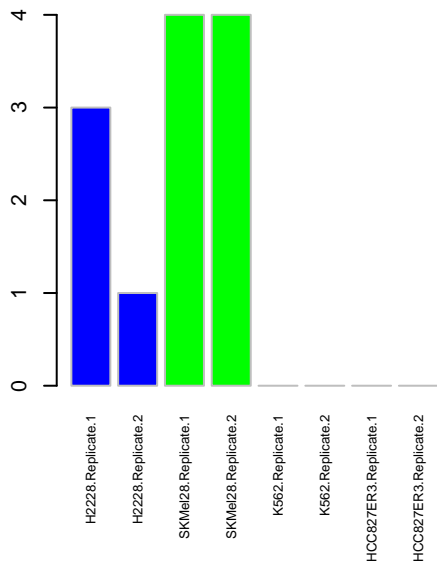
Kinome INSR
