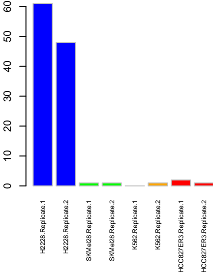
NWK EPHA1
