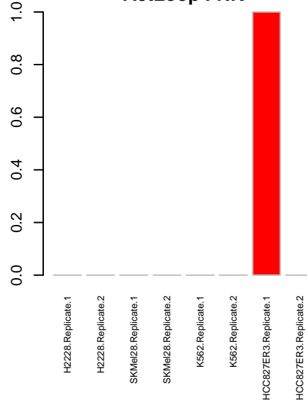
ActLoop FRK
