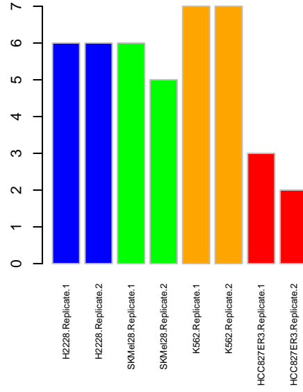
ActLoop FYN
