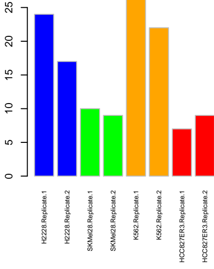
PSP MAP3K5
