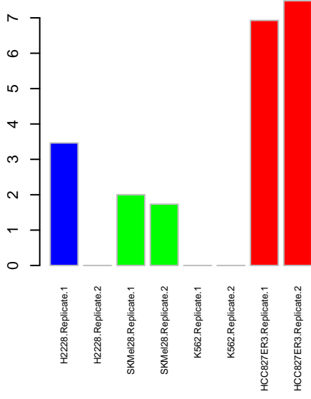
InKA EPHA3
