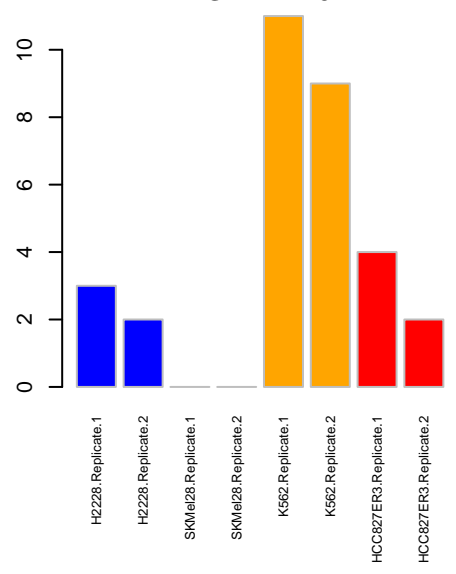
PSP ZAP70
