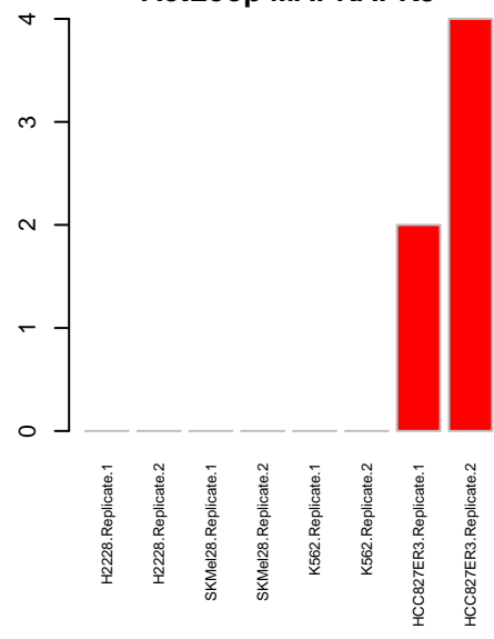
ActLoop MAPKAPK3
