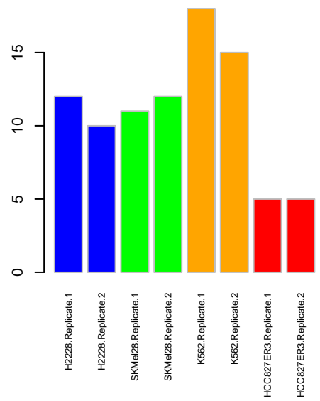
Kinome DYRK1B
