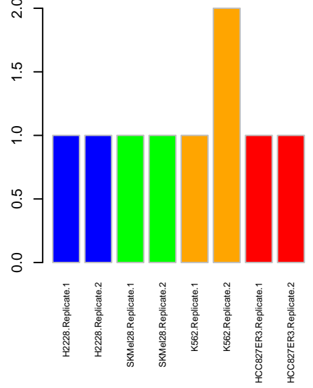
Kinome FGR
