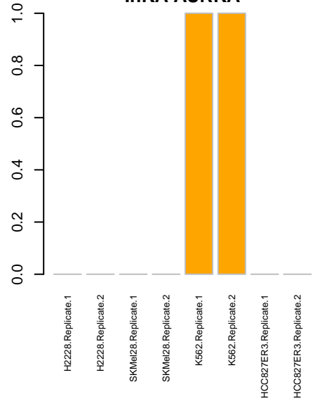
InKA AURKA
