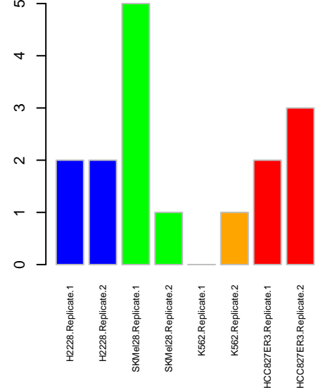
Kinome MAPK9
