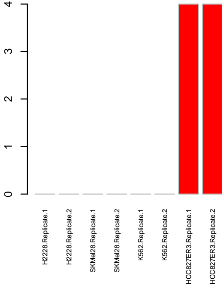
Kinome ERBB3
