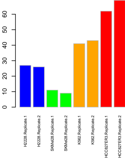
NWK ITK
