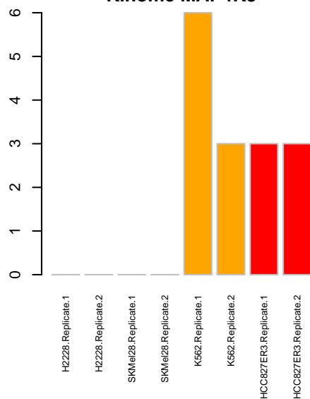
Kinome MAP4K3
