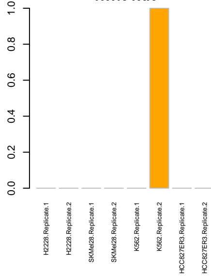
NWK TXK
