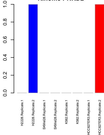
Kinome PRKD2
