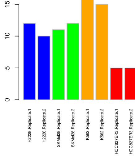
ActLoop DYRK1A
