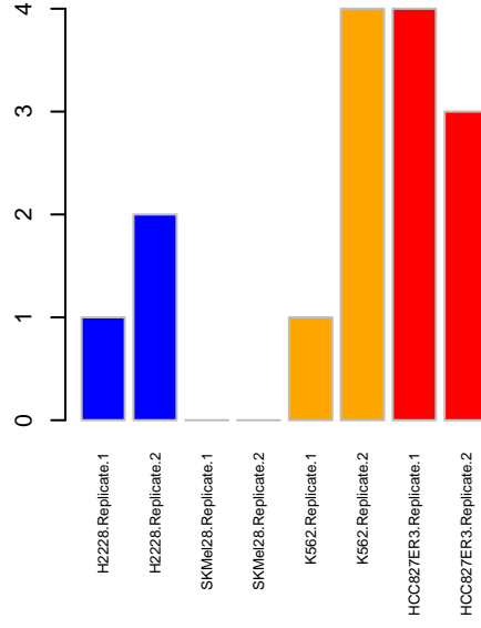
PSP AKT1
