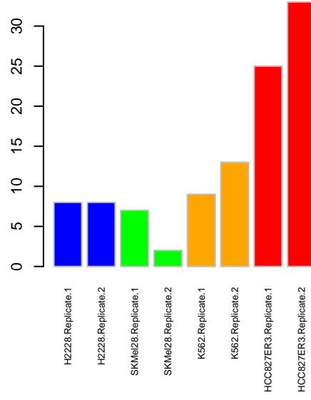
NWK MAP2K4
