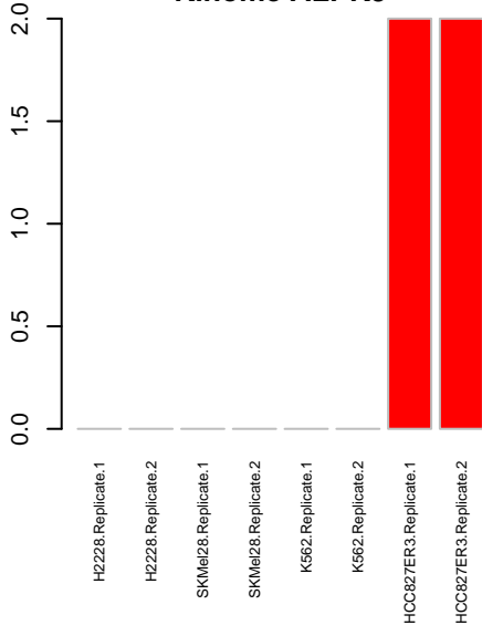
Kinome ALPK3
