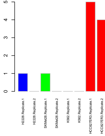
PSP FGFR3
