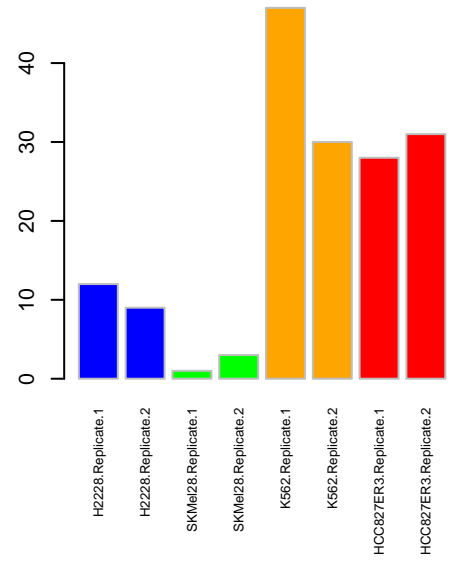
NWK PDGFRB
