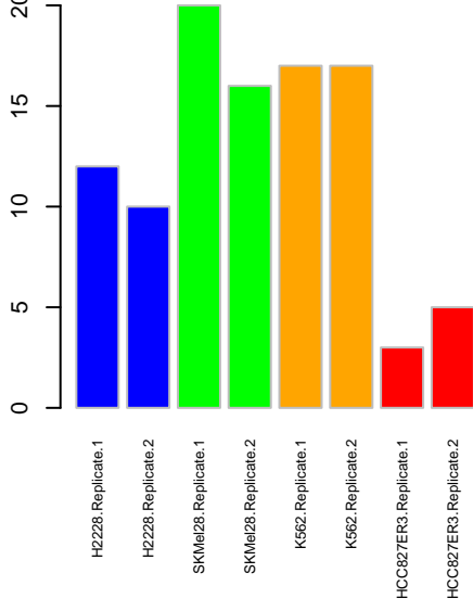
PSP MAP2K2
