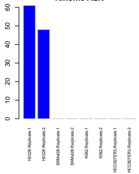
Kinome ALK
