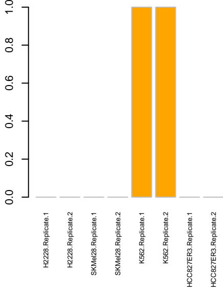
Kinome AURKB
