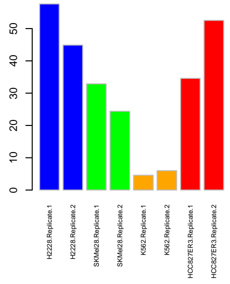
InKA PTK2
