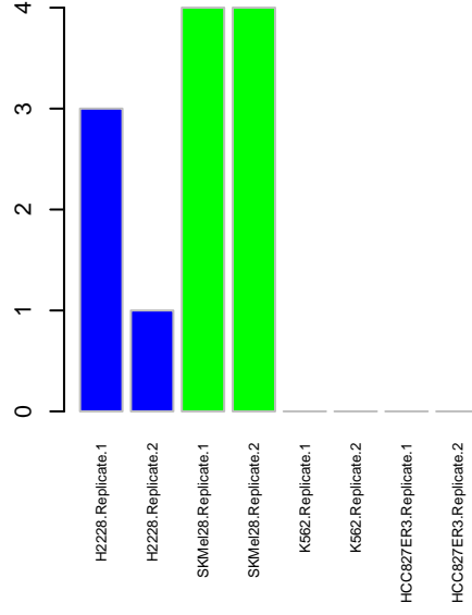
ActLoop IGF1R
